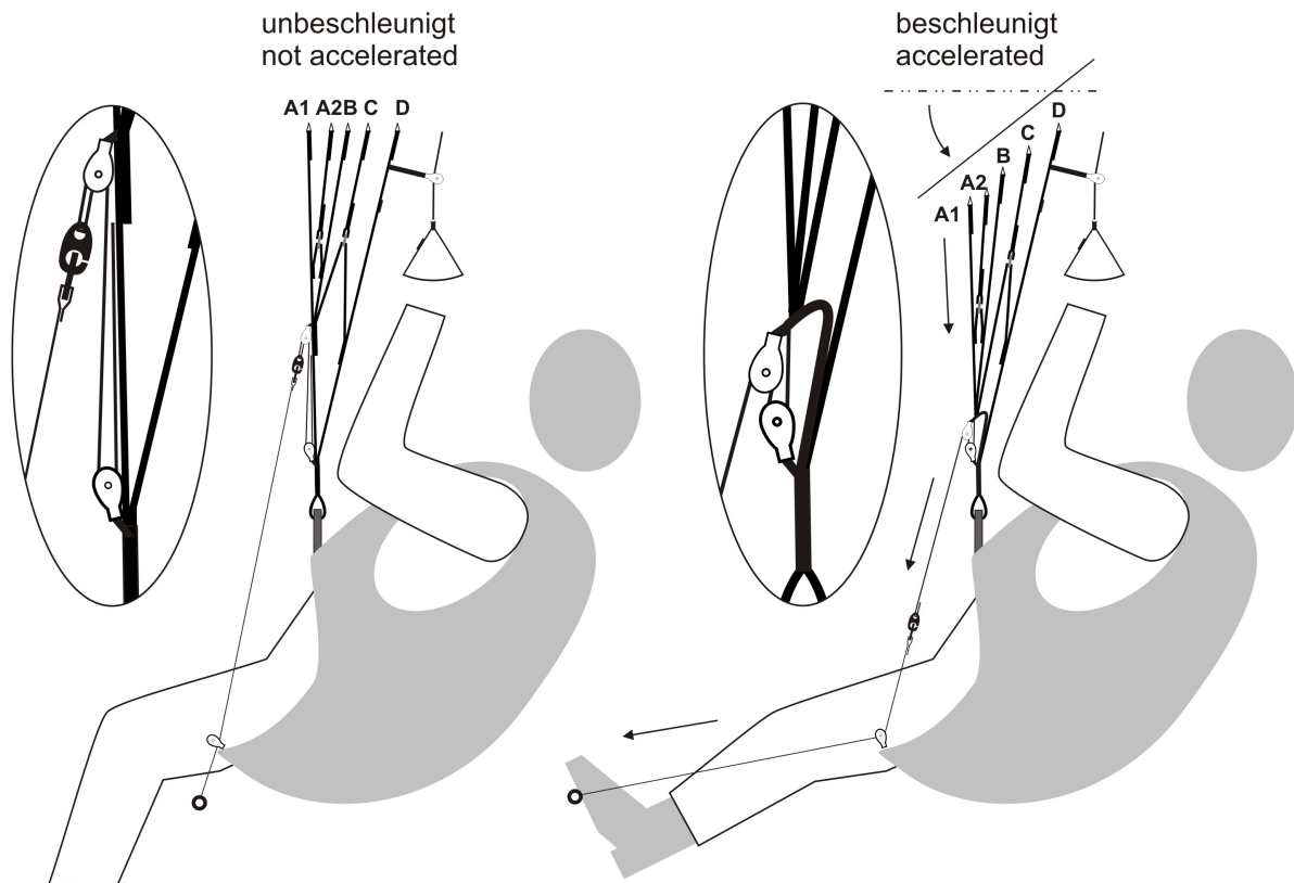
Bild 2: Funktionsweise Fußbeschleuniger MISTRAL 6
