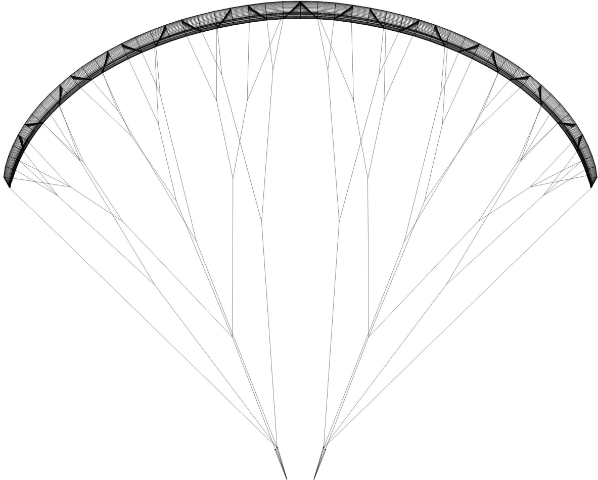
Bild 1: Gittermodell MISTRAL 6 (Frontansicht)
