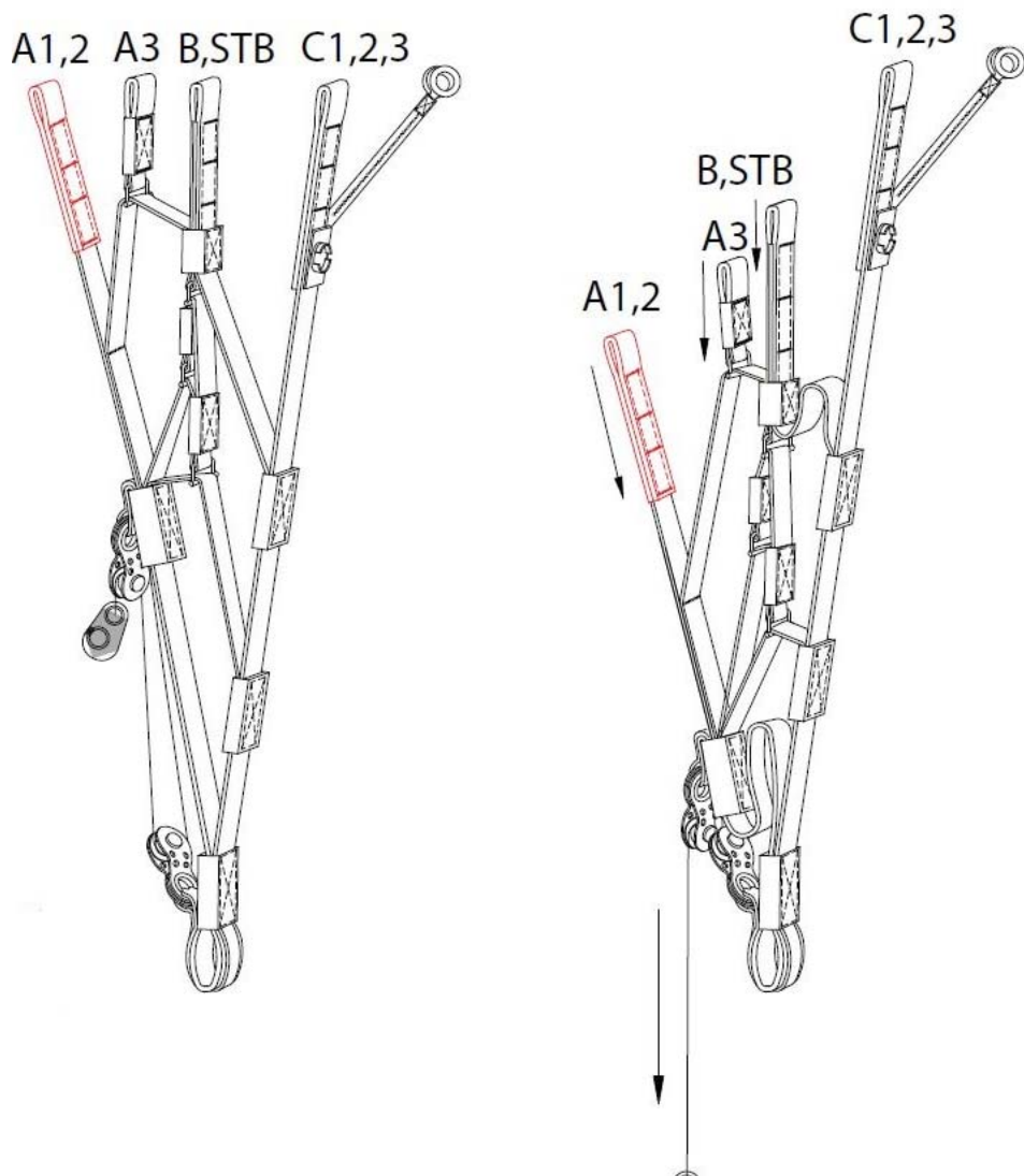
Abbildung 5: GTO 2 Tragegurte (Trimmstellung und voll beschleunigt)
