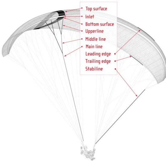
Abbildung 4: Übersichtszeichnung
