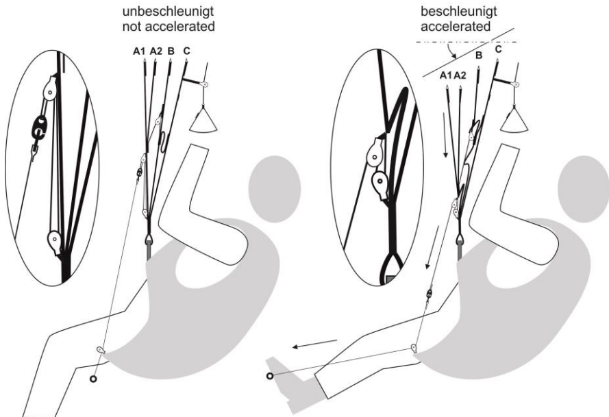
Abbildung 5: Funktionsweise Fußbeschleuniger Sensis
