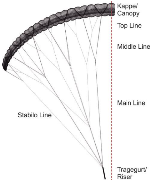
Abbildung 1: Gittermodell Sensis
