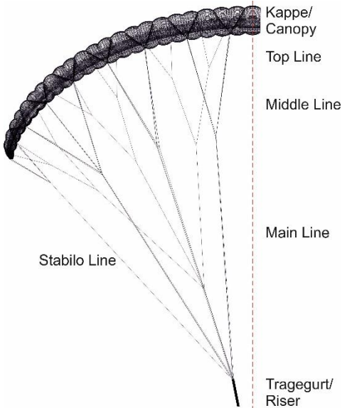
Abbildung 1: Gittermodell Nexus
