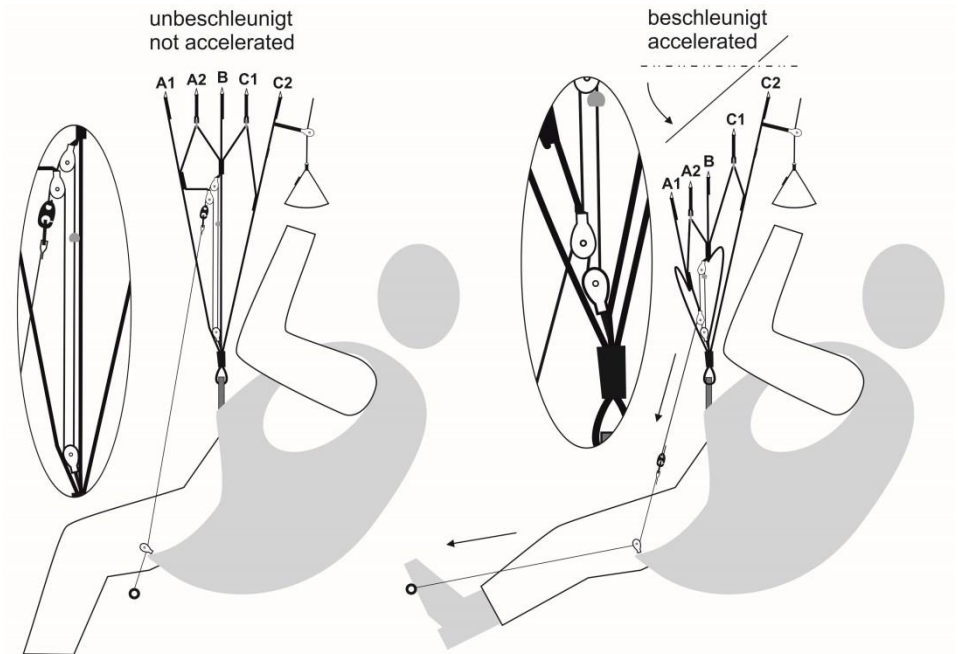
Abbildung 5: Funktionsweise Fußbeschleuniger Nexus
