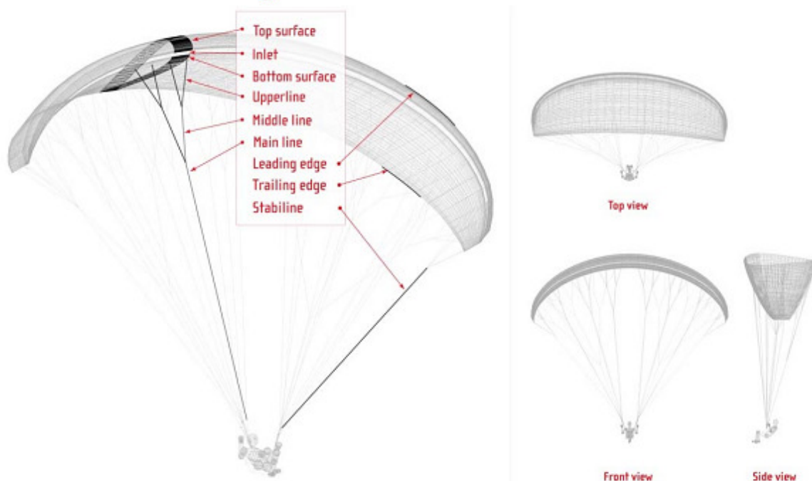
Abbildung 4: Übersichtszeichnung
