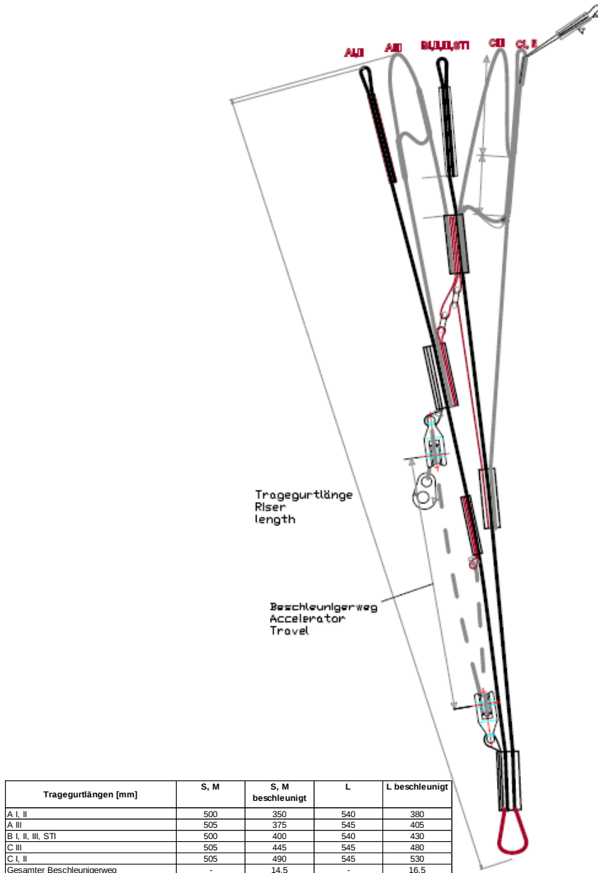
Abbildung 4: Tragegurte des UP Lhotse
