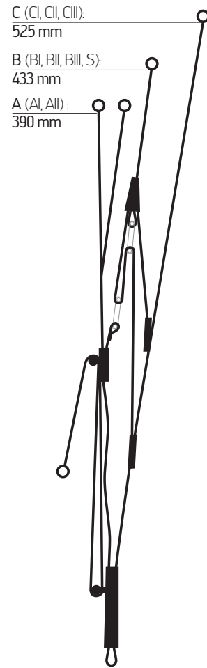
Beschleunigter Flug
