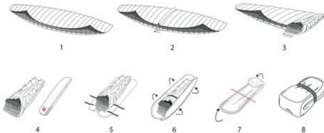
Abbildung: Richtiges Packen des Pegasus 2
