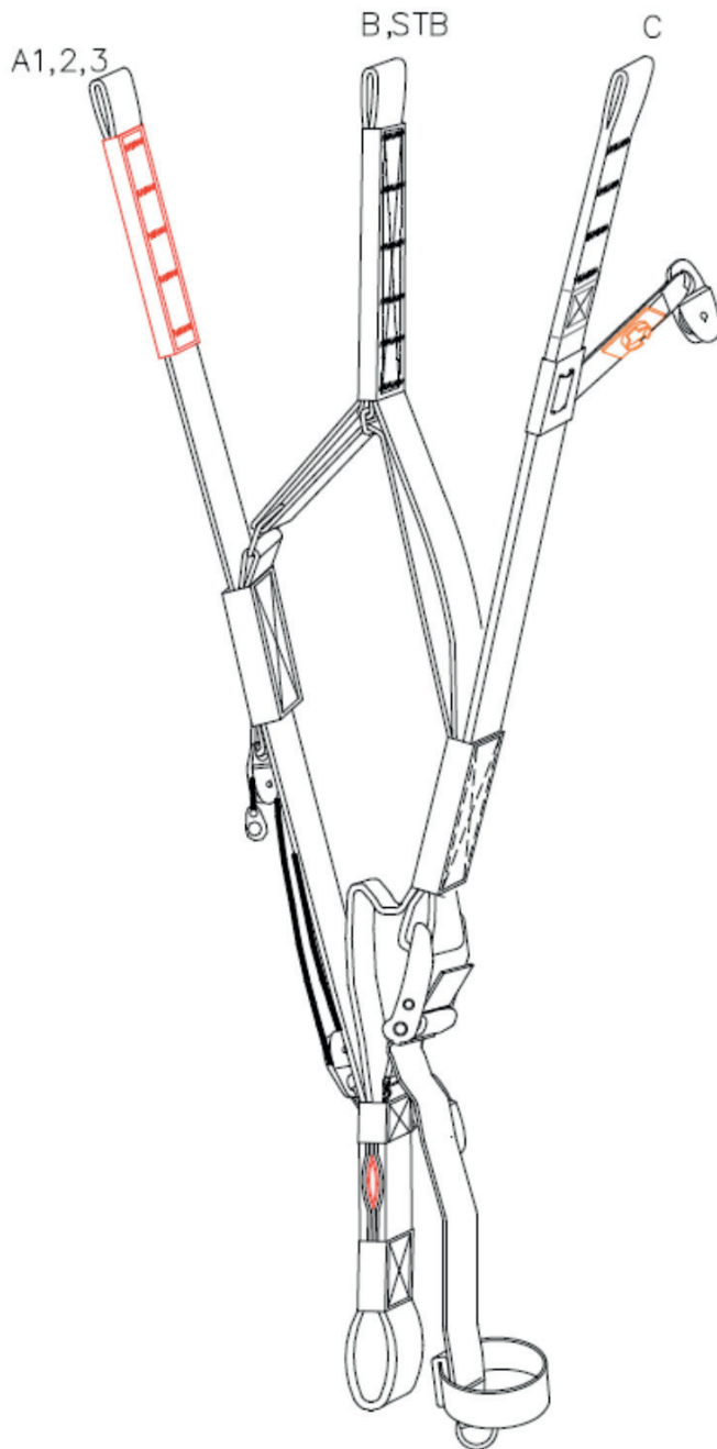
Abbildung: Standard-Tragegurte des Pegasus 2
