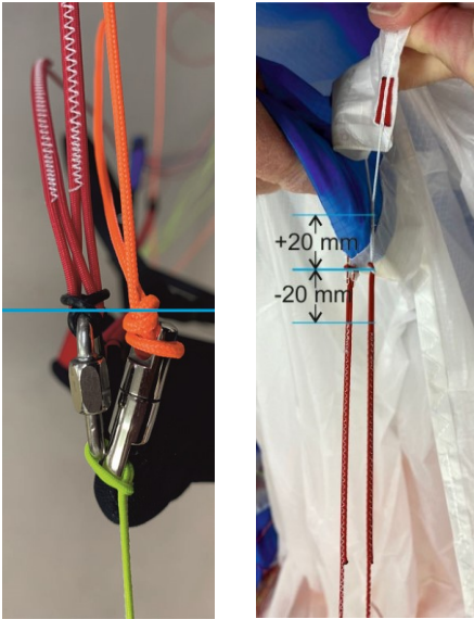
Abb. 10. Meßpunkte für Bremsleinen Schnellcheck
