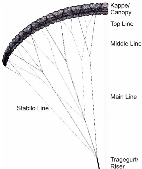
Abb. 1. Gittermodell ARCUS 2 RS
