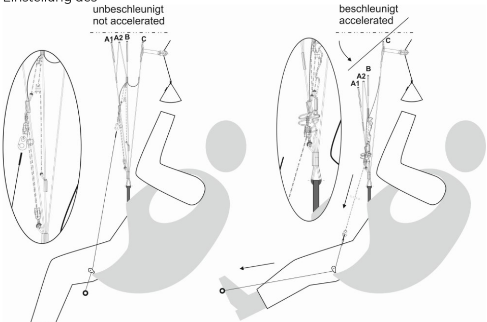
Abb. 1. Funktionsweise Fußbeschleuniger ARCUS 2 RS
