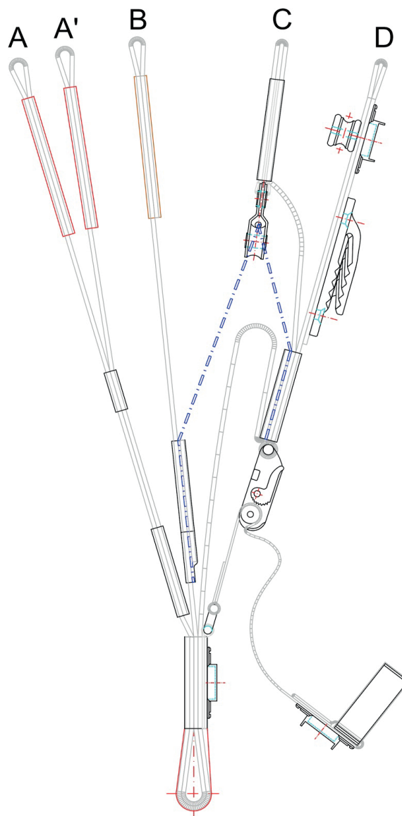
Abbildung: Tragegurt mit 20 mm Gurtband
