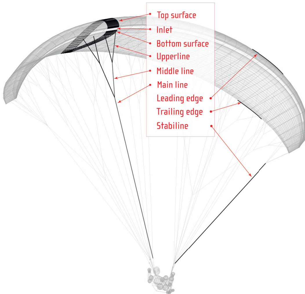
Abbildung: Allgemeine Übersichtszeichnung und Beschreibung der Gleitschirmbauteile
