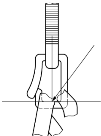
Bild 3 — Oberer Messpunkt am Gurtzeug
