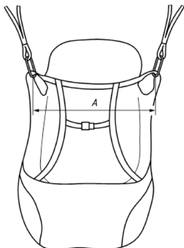
Bild 5 — Breite der Befestigungspunkte des Gurtzeugs
