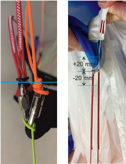
Abb. 9. Meßpunkte für Bremsleinen Schnellcheck
