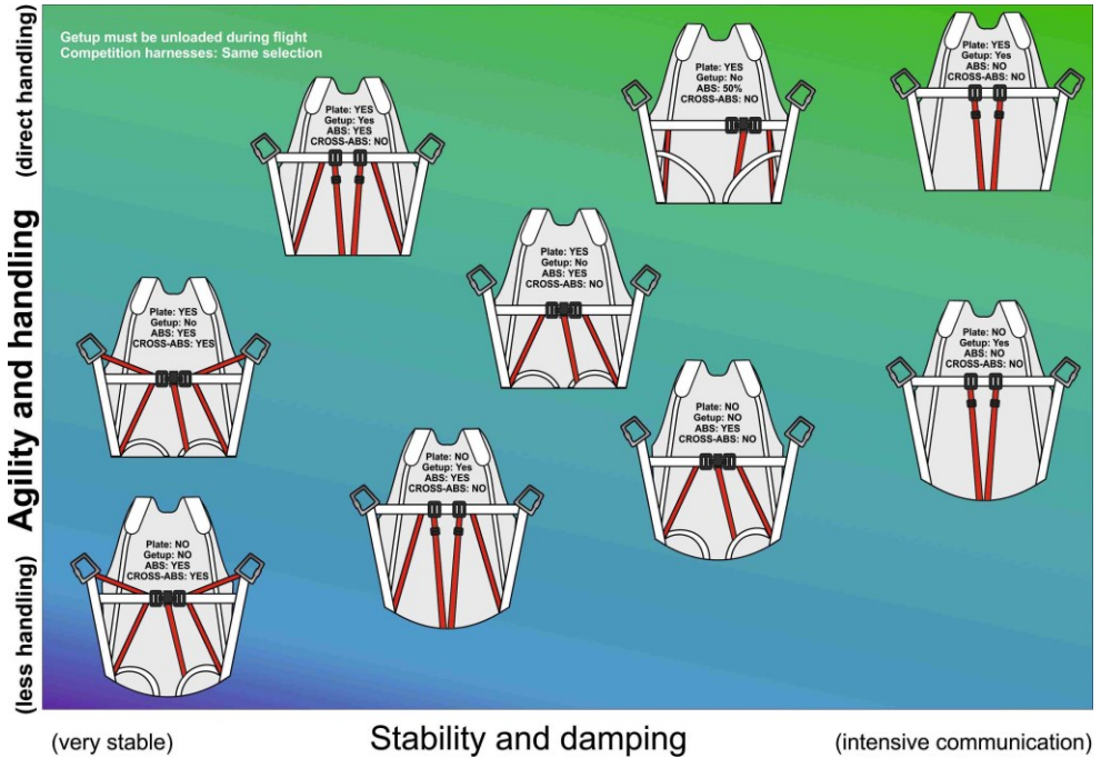
Abb. 7. Übersicht verschiedene Gurtzeuggeometrien und deren Dämpfung
