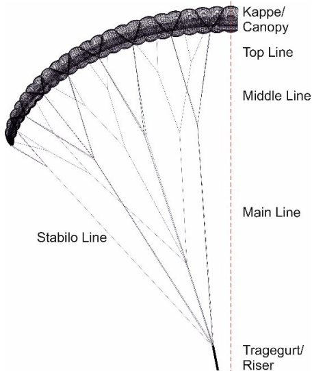
Abb. 1. Gittermodell SERAC RS
