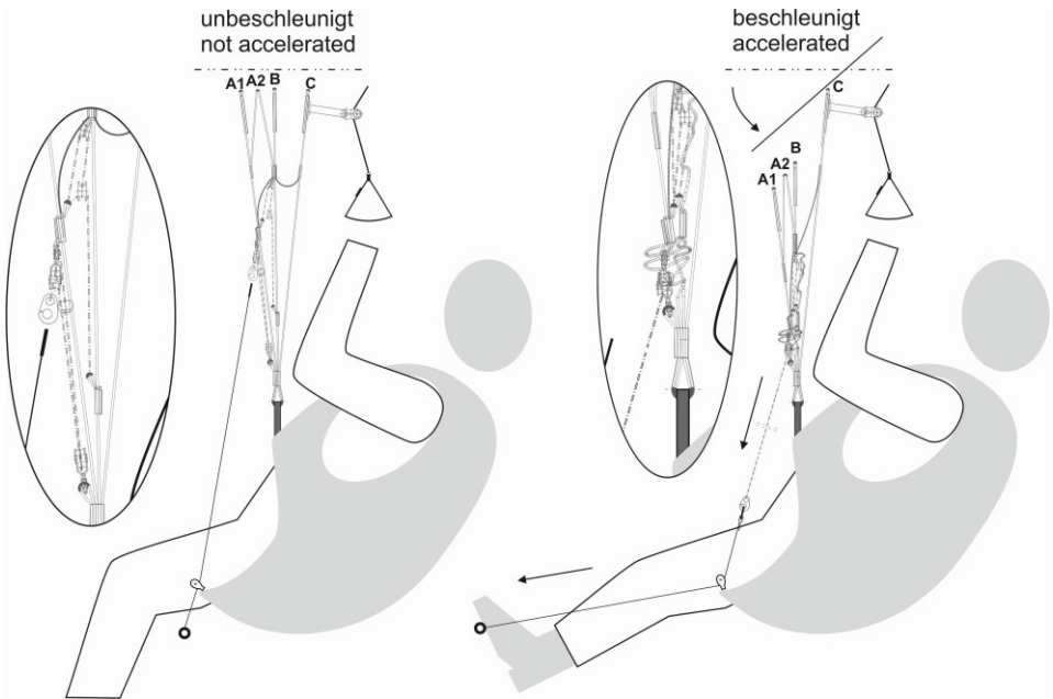
Abb. 6. Funktionsweise Fußbeschleuniger SERAC RS
