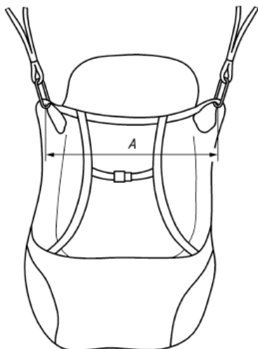
Bild 5 — Breite der Befestigungspunkte des Gurtzeuges
