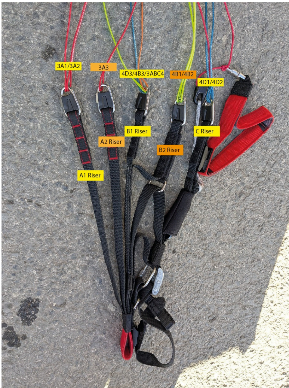
Trimmer geschlossen
