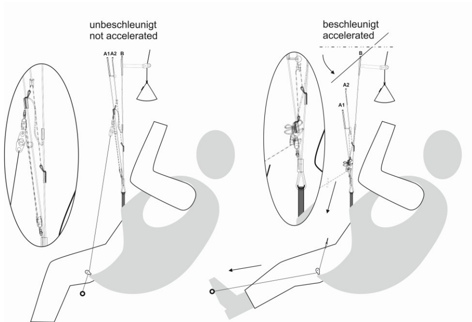
Abb. 3. Funktionsweise Fußbeschleuniger SPHERA 2 RS
