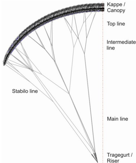
Abb. 1. Gittermodell SPHERA 2 RS
