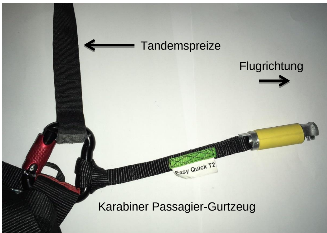
Abbildung 4.1: Detailsicht der Einhängung am linken Karabiner des Passagier-Gurtzeuges
