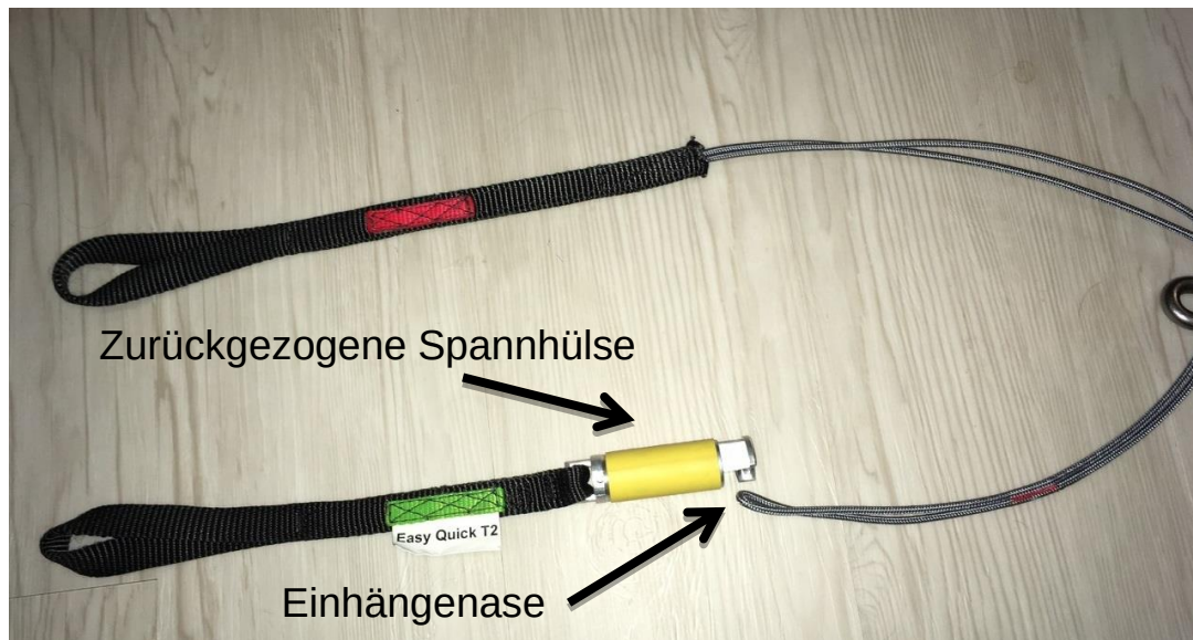
Abbildung 5.1: Spannhülse zurückgezogen
